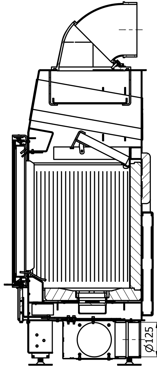
A-A ( 1 : 8 )
